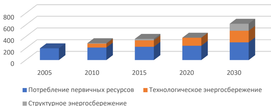
Рис. 1. Энергетическая стратегия Украины на период до 2030 года: Прогноз динамики потребления первичных ресурсов, уровней структурного и технологического энергосбережения до 2030 года, млн. т у.т. (базовый сценарий). Показатели за 2005 г. во всех раздела
